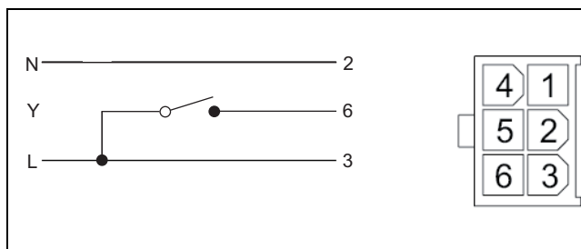
Afb. 23 Molex-connector
