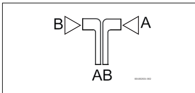
Afb. 24 Hydrauliek voor omschakelventiel TW1
