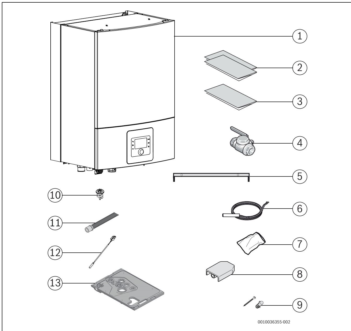
Afb. 2 Meegeleverde onderdelen
