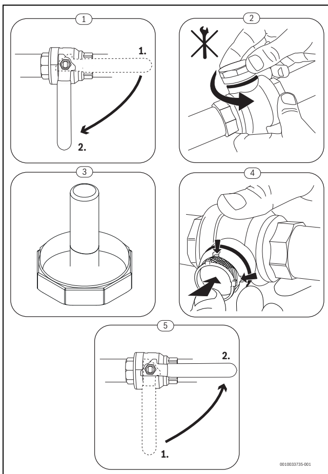
Afb. 19 Filterreiniging
