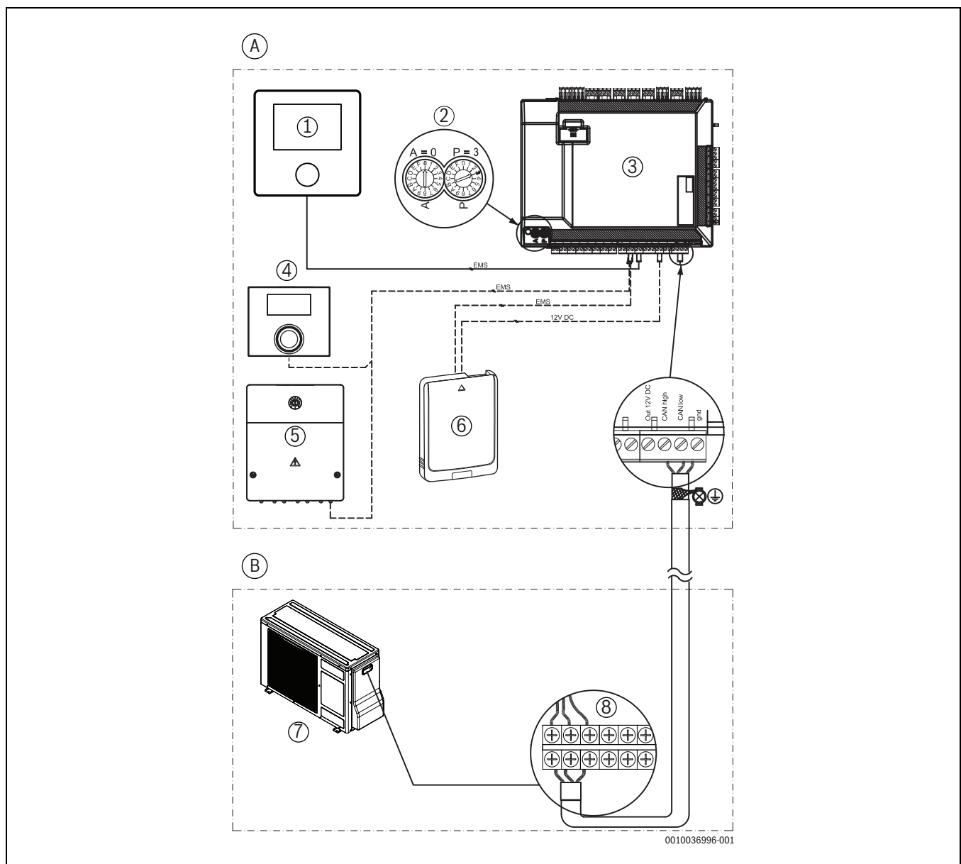
Afb. 38 CAN en EMS aansluitingen
