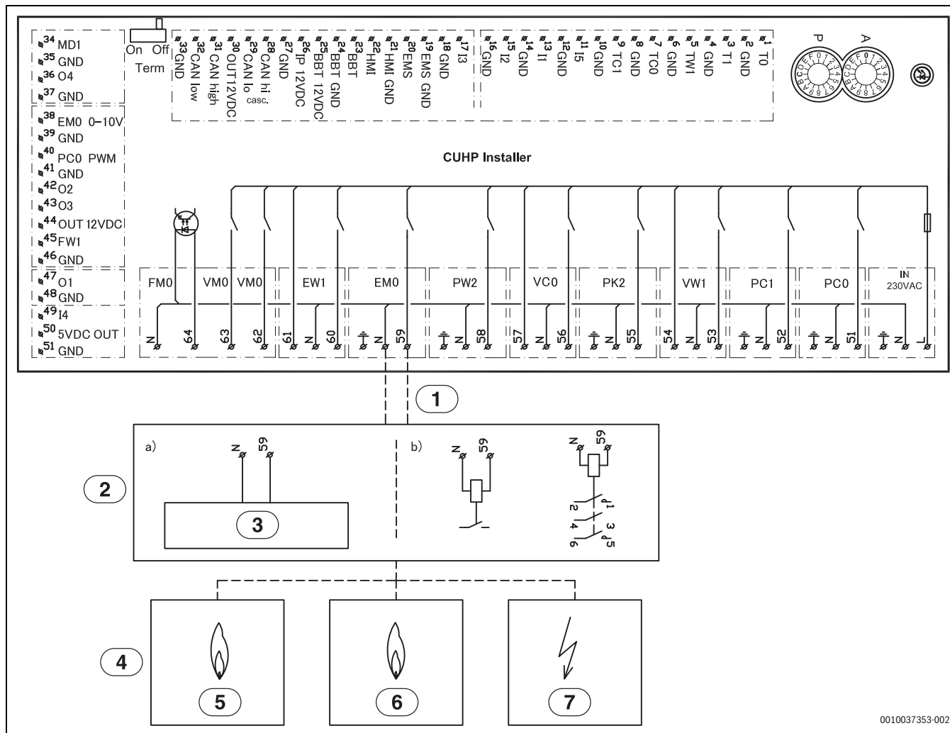
Afb. 14 Installatieprintplaat elektrische schema start/stop
