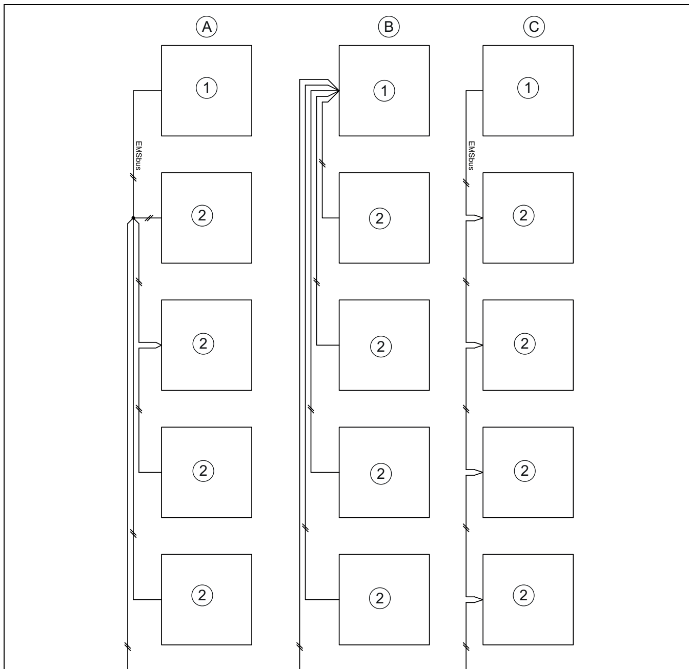
Afb. 41 Aansluitalternatieven voor EMS-bus
