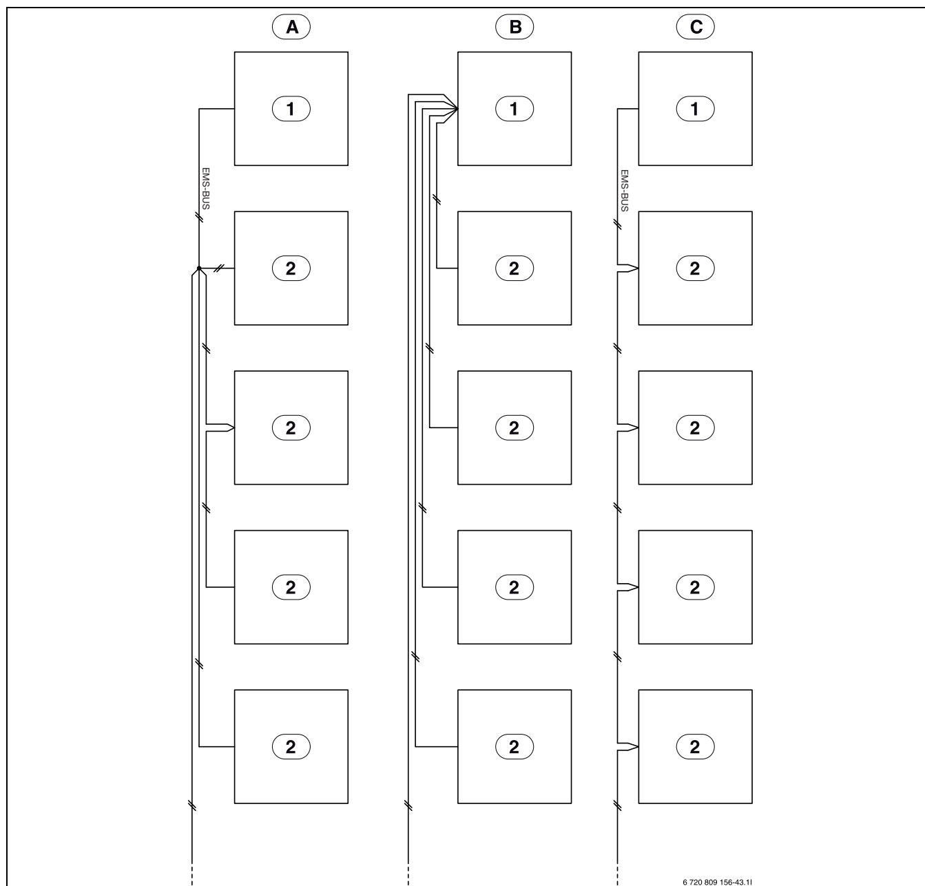
Afb. 37 Alternatieve aansluiting op de EMS-BUS
