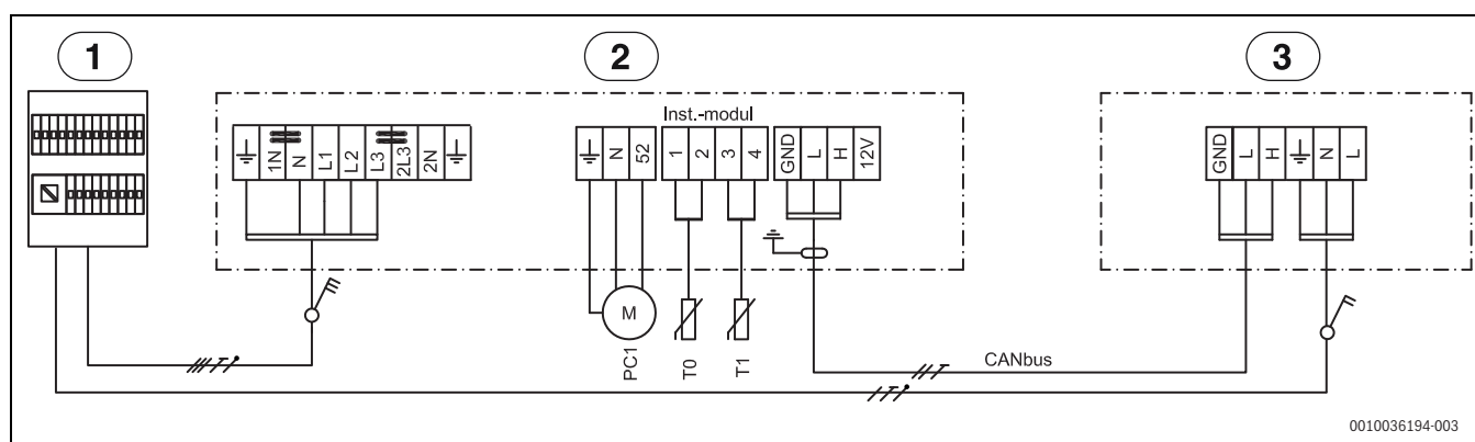
Afb. 35 Elektrisch schema 5,85 kW 400 V 3 N~
