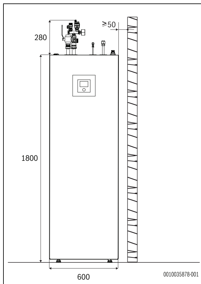
Afb. 5 Afmetingen (mm)
