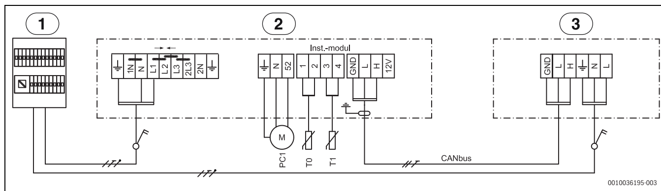
Afb. 34 Elektrisch schema 5,85 kW 230 V~
