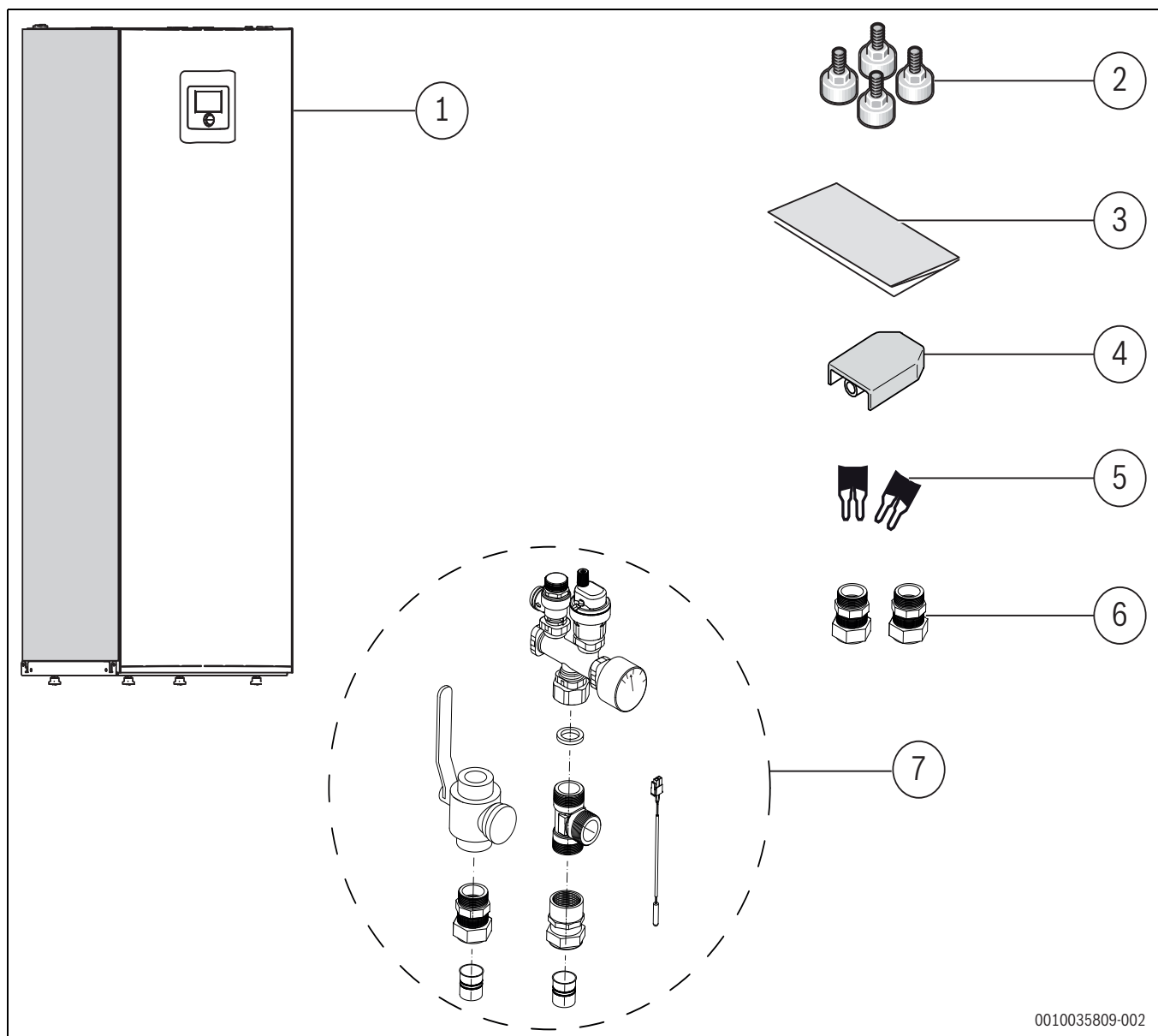
Afb. 2 Meegeleverde onderdelen
