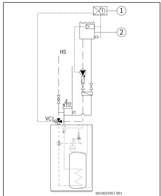
Afb. 22 Zwembadinstallatie
