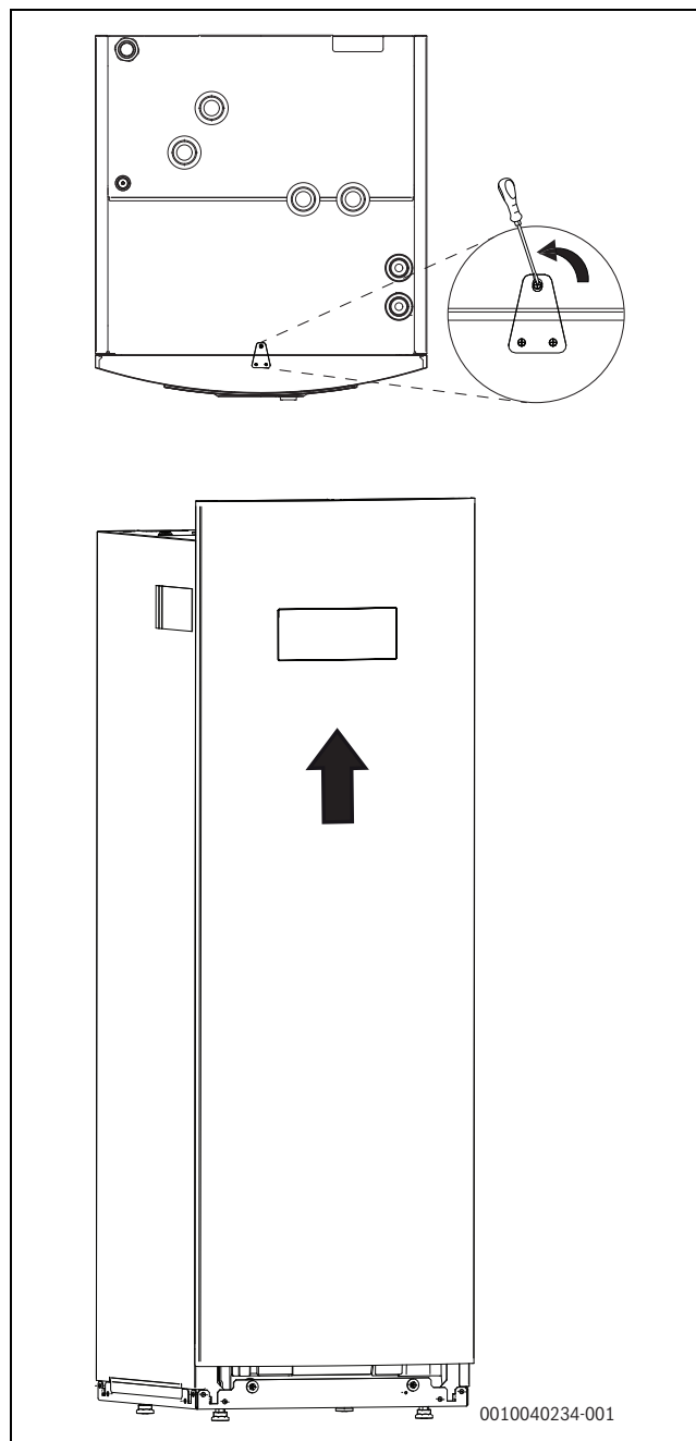
Afb. 7 Verwijderen van het frontpaneel van de binnenunit
