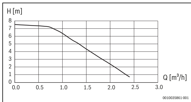
Afb. 25 Capaciteitscurve van de primaire circulatiepomp (PCO)
