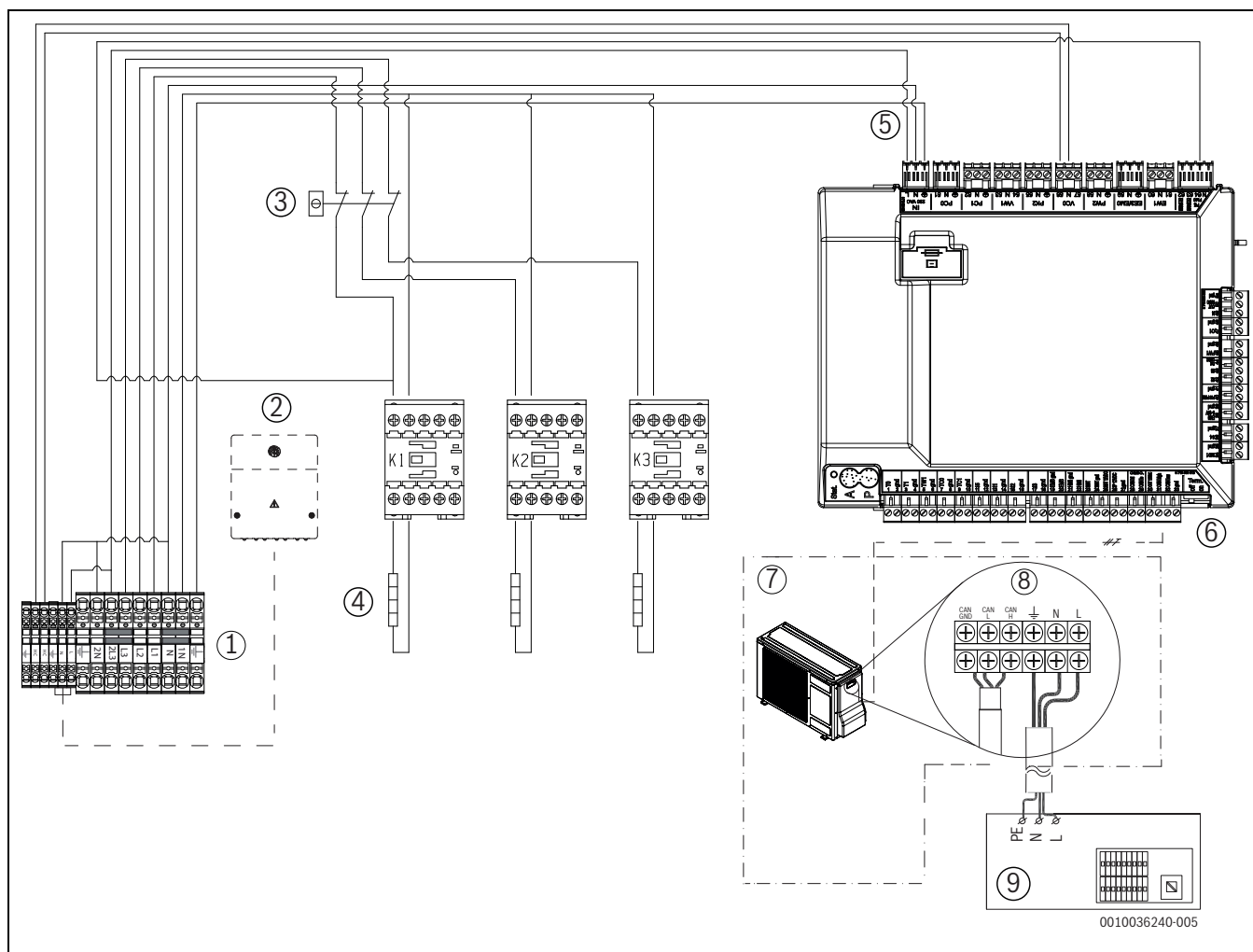
Afb. 36 400 V 3N~ binnenunit met 230 V~ buitenunit
