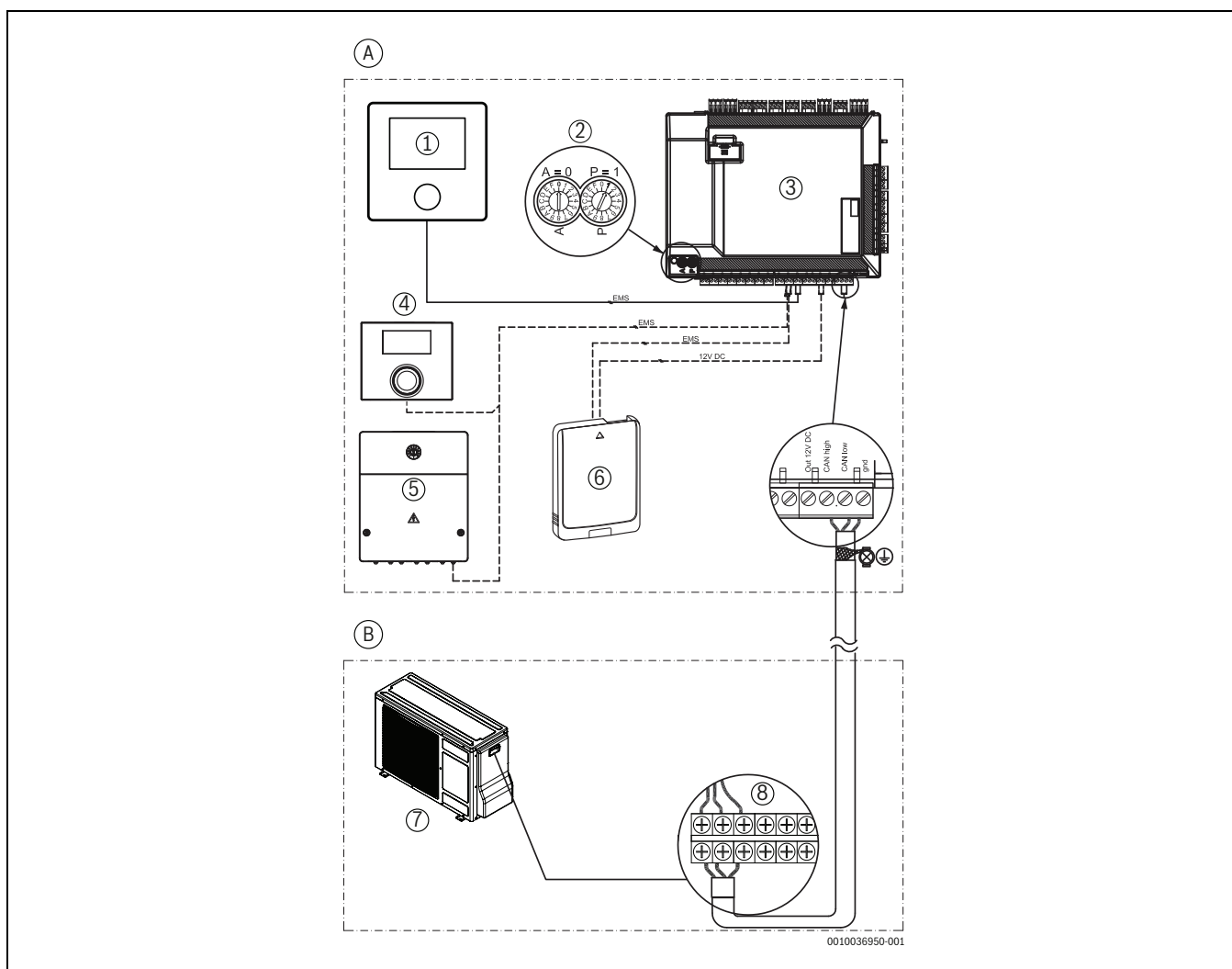
Afb. 33 CAN en EMS aansluitingen
