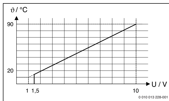
图2 0-10 V 信号 ( U 单位为V) 和要求的出水温度 \theta (单位为 °C, 以最低出水温度至最高出水温度的范围为基准 [基本设置 20 °C 至 90 °C]) 之间的线性关系
