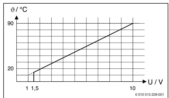
Fig. 2 Relación lineal entre señal 0-10V (U en Volt) y la temperatura de impulsión requerida \theta (en °C relación del sector de la temperatura mínima de impulsión hasta una temperatura máxima de impulsión [Ajuste de fábrica 20 °C hasta 90 °C])
