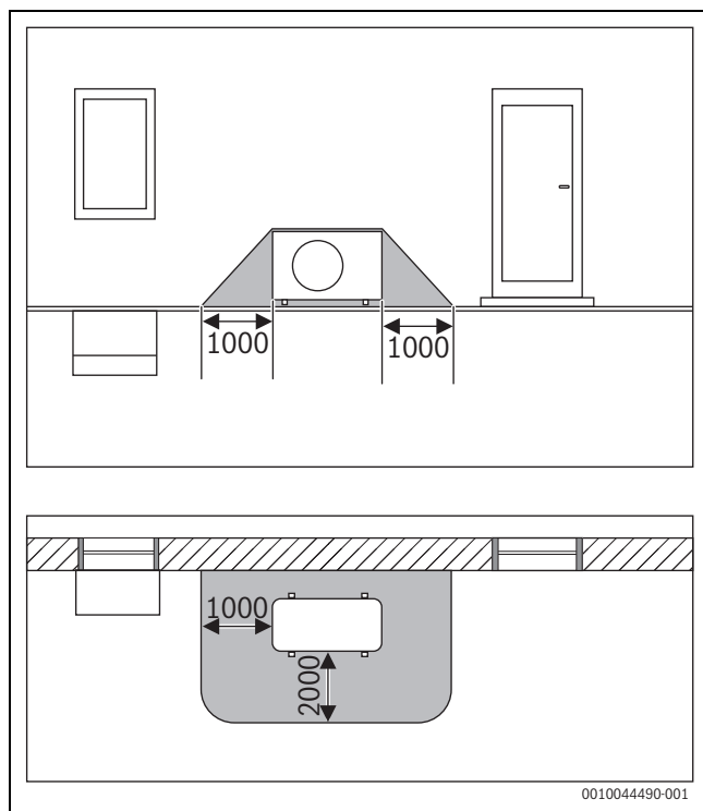
Joon. 1 Ohupiirkond, seinä ääres põrandal seisev välisseade (mõõdud mm-tes)
