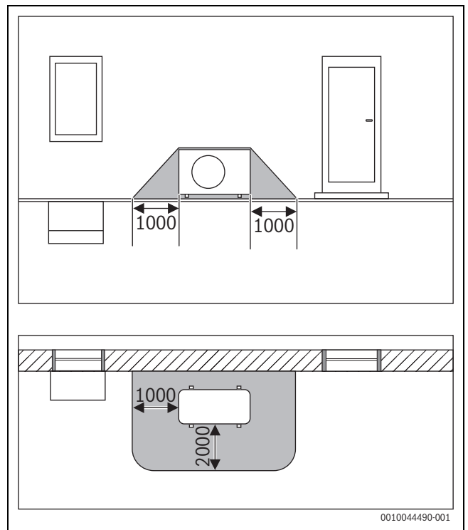
Sl.1 Varnostno območje, talna zunanja enota na steni (mere v mm)
