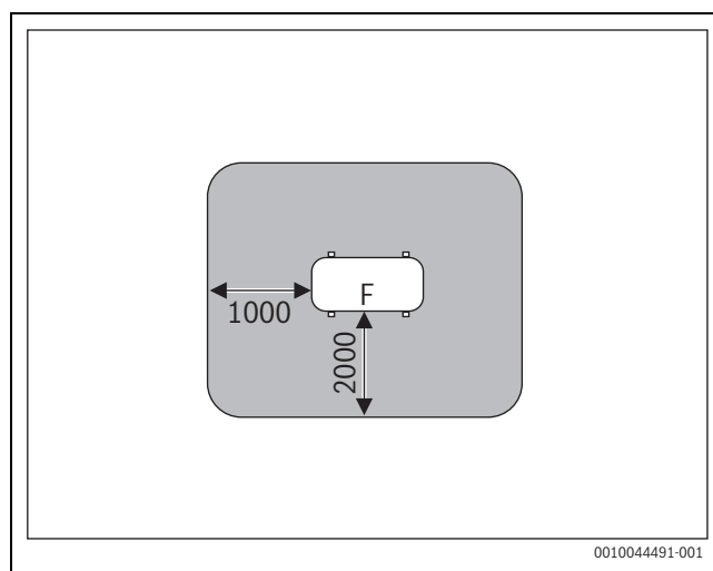
Att. 2 Aizsardzības zona, uzstādot iekārtu uz zemes uz gruntsgabala vai jumta (izmēri mm)
