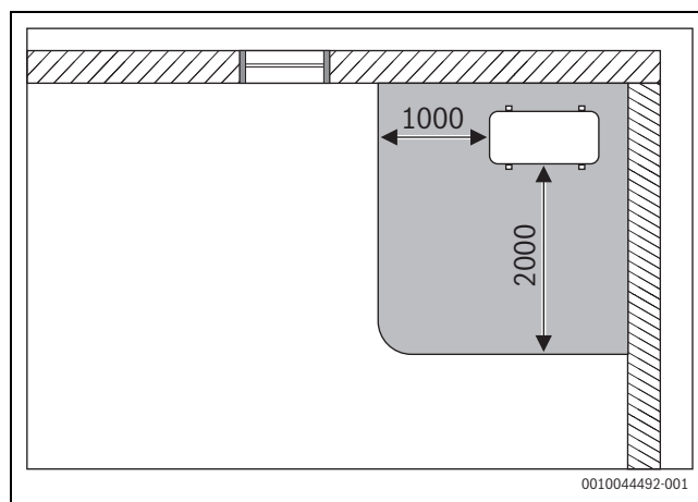
Joon. 3 Ohupiirkond, nurgas põrandal seisev välisseade (mõõdud mm-tes)
