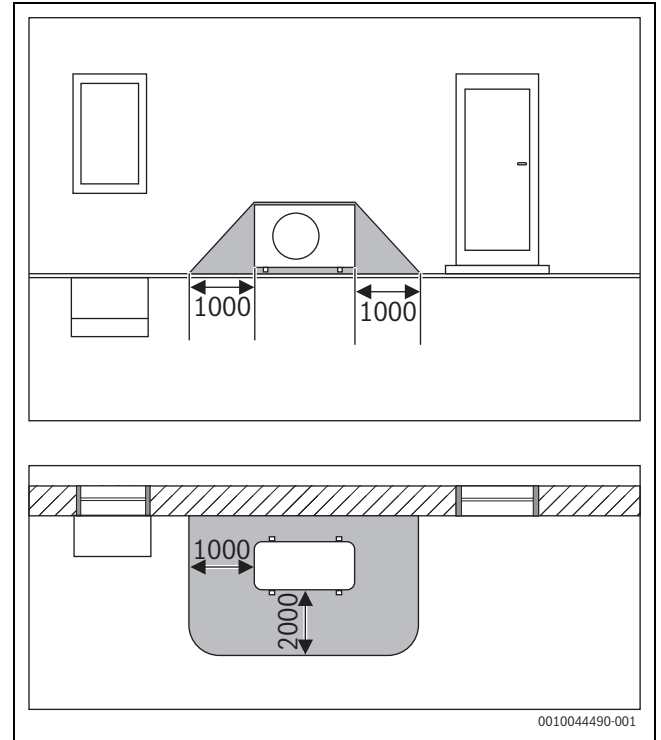
Σχ. 1 Προστατευμένη περιοχή, εξωτερική μονάδα τοποθετημένη στο δάπεδο σε τοίχο (διάσταση σε mm)
