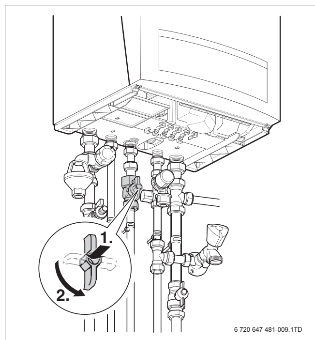
Afb. 3 Gaskraan
