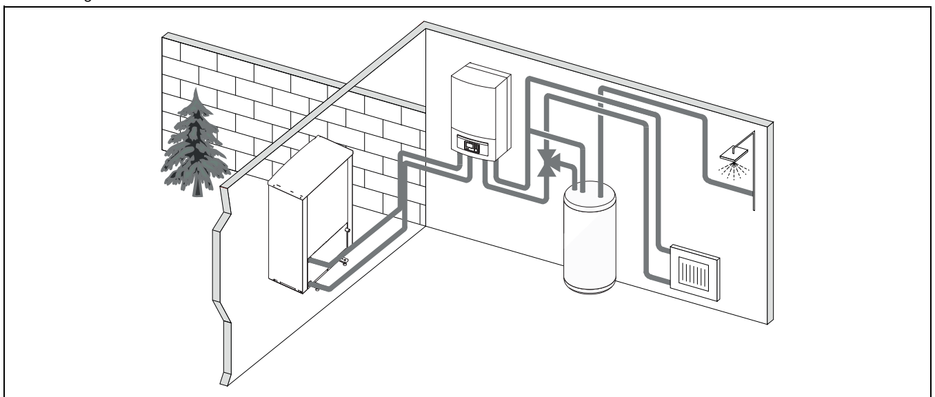
Afb. 3 Warmtepomp ODU Monoblock A/W, binnenunit IDU Monoblock E met elektrische bijverwarming en externe boiler
